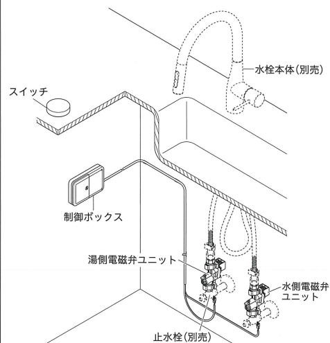
〈遠隔スイッチセット取り付け例〉
